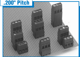
ESTT Multi-tier . . . . . Pages 74-75 24A / 300V
