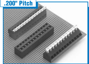
SCM Spring-Clamp . . . . . Page 82 20A / 300V
