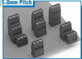
ESMT Multi-tier . . . . . Pages 72-73 17.5A / 300V
