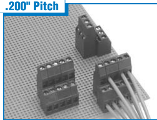
EL2M Right-Offset . . . . . Page 69 20A / 300V
