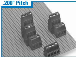
EL1M /2M /3M . . . . . Page 68 20A / 300V
