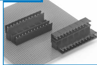
ELFD 2-Tier Offset H/V . . . . Page 37 12A / 300V
