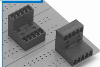
ELVD 2-Tier Offset H/V . . . . Page 24 12A / 300V
