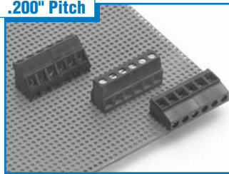
ELM Standard Profiles . . . Page 64 15A / 300V
