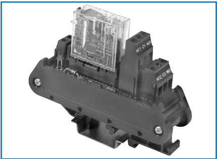
IRL Relay Module. . . . . Page 98
