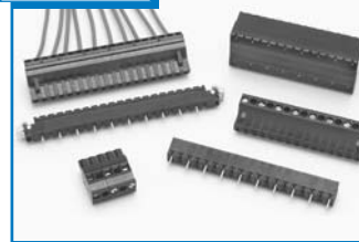
ELLP, ELLT, ELLF, ELLK . . . Page 55 15A / 600V
