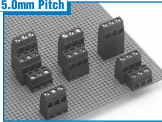
ESLT Multi-tier . . . . . Pages 70-71 13.5A / 300V
