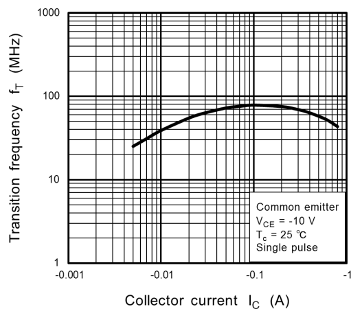
Fig. 7.5 f_T - I_C
