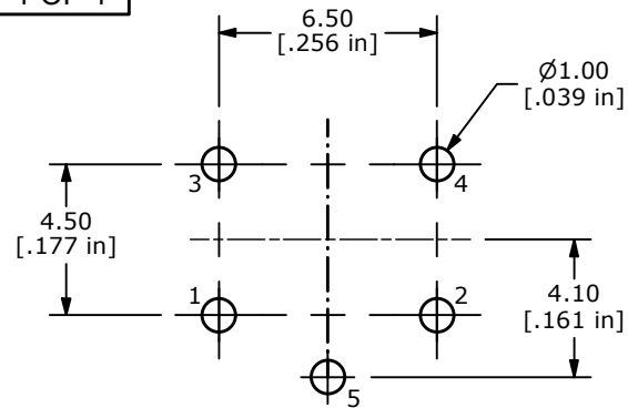
P.C. LAYOUT
