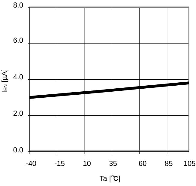
Fig.24 T_a - I_{EN}
