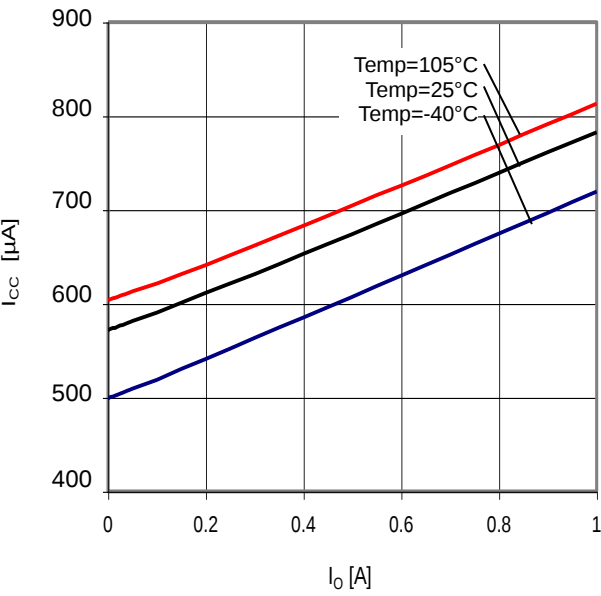
Fig.30 I_o-I_{cc}
