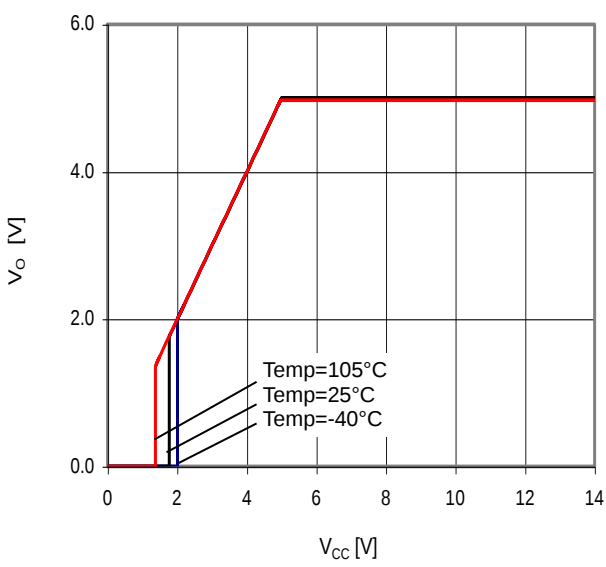
Fig.27 V_{CC}-V_o ( I_o=0\text{mA} )
