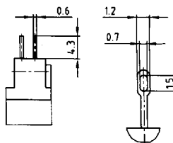
Solder lug
