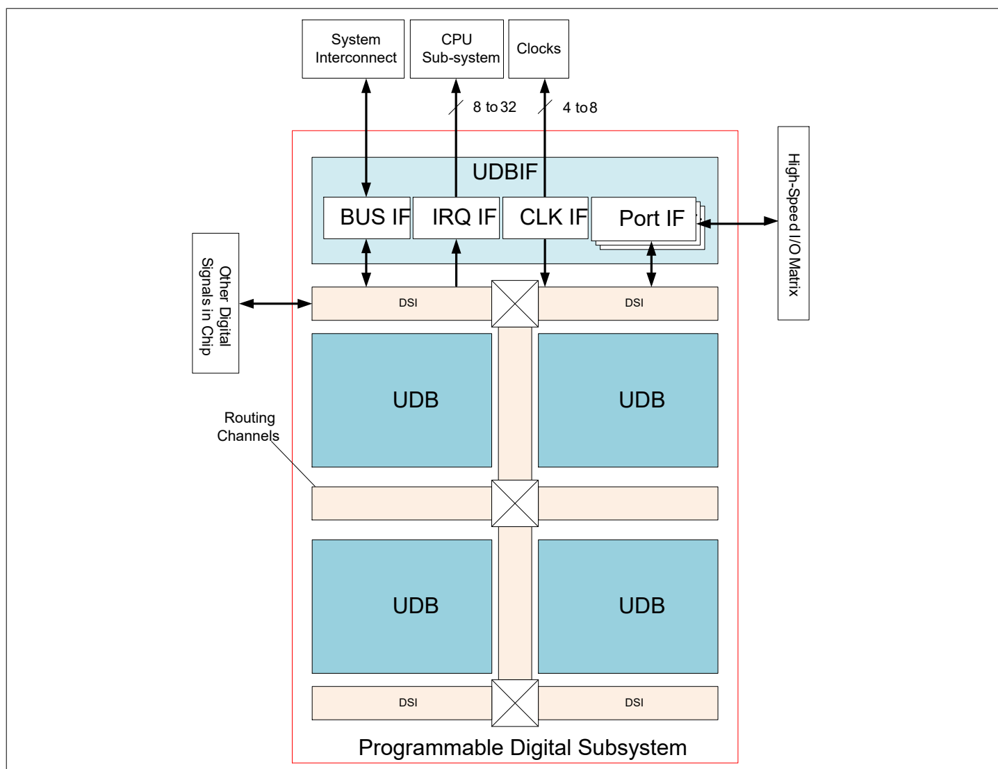
Figure 4 UDB array
