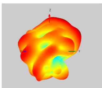
2400MHz
