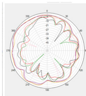
YZ-PLANE
