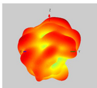
2450MHz
