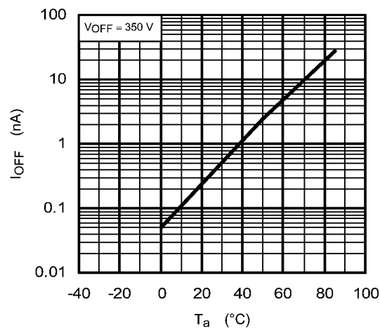
Fig. 16.9 I_{OFF} - T_a
