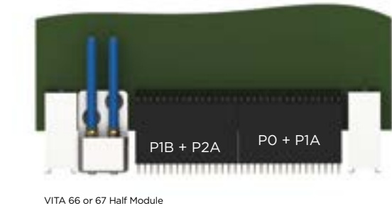
VITA 66 or 67 Half Module
