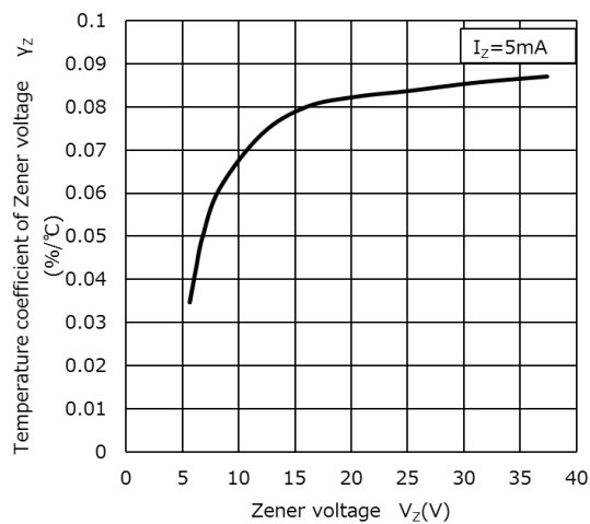
\alpha_Z - V_Z
