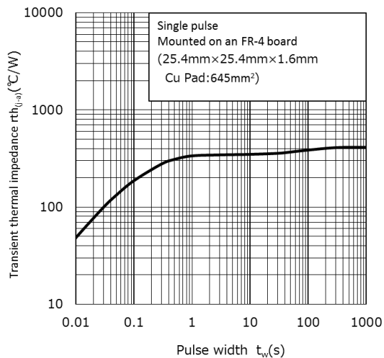
r_{th(j-a)} - t_w
