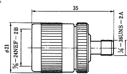
HRM-508(40)
