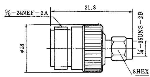
HRM-507(40)
