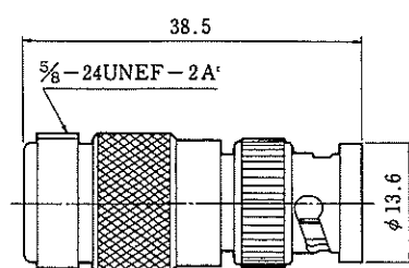
UG-349/U(40)
