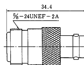
NJ-BNCJ(40)
