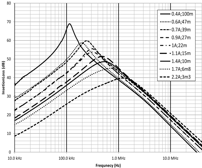
RN 218
