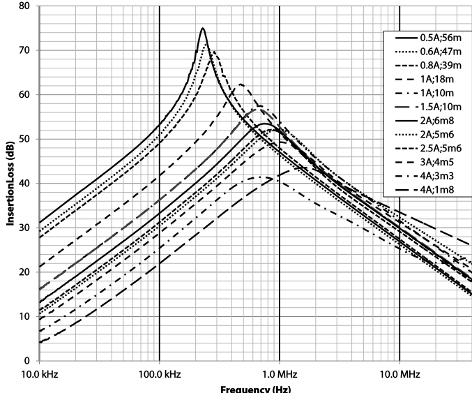
RN 122, RN 222
