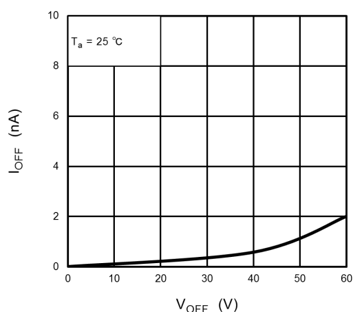
Fig. 12.1.10 I_{OFF} - V_{OFF}
