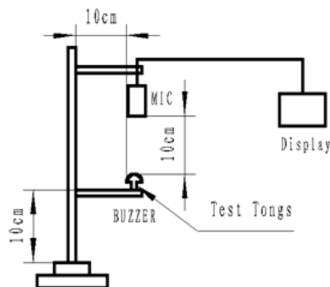
Test Equip
