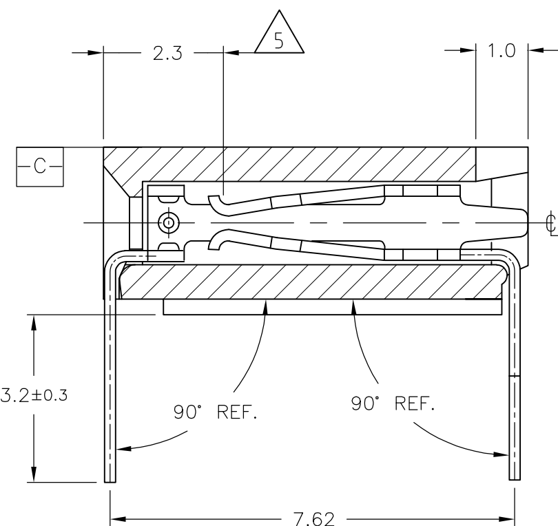
SECTION A-A
