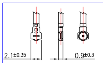
Detail A Scale: 1:3
