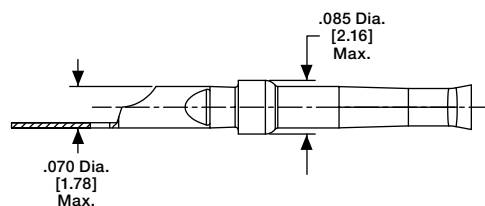
Socket
