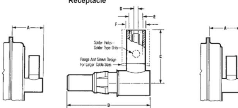
Receptacle
