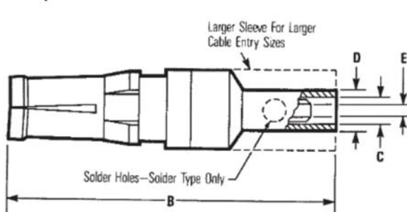
Receptacle
