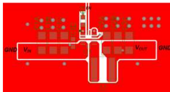
Top Layer
