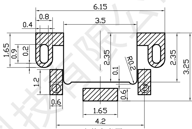
安装参考图
