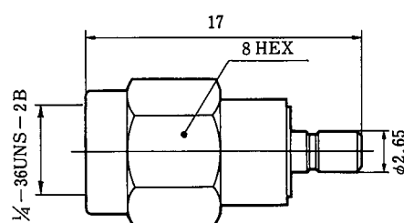
HRMP-PO6J CL311-0172-4
