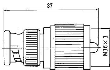
BNCP-MP CL311-0062-6
