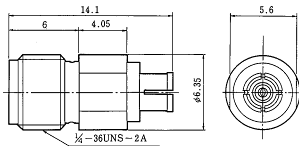
HRMJ-S.FLP CL311-0218-3
