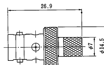
BNCJ-PODP CL311-0160-5
