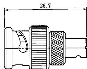
BNCP-MSSP CL311-0107-2
