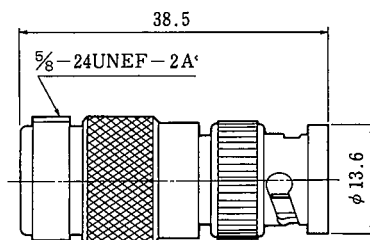
UG-349/U CL311-0004-0
