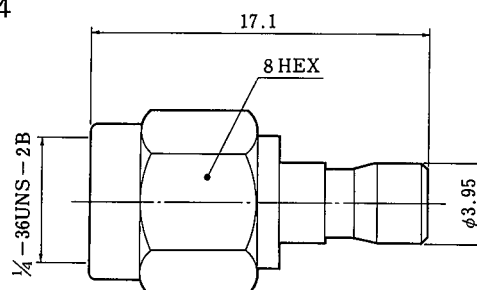
HRM.P-POD.J CL311-0177-8
