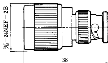
SP-BNCP CL311-0055-0
