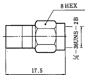
HRMP-POD1J CL311-0253-4
