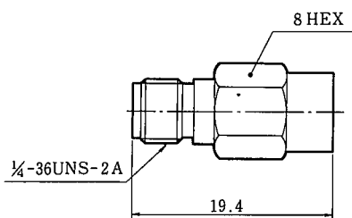
HRMJ-POD1P-1 CL311-0254-7
