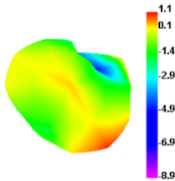
2100.000MHz E1
