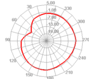
2100.000MHz E2
