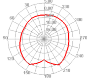
2650.000MHz E1
