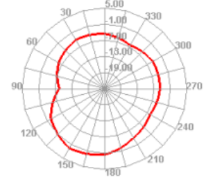
2450.000MHz E2
