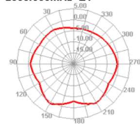
2350.000MHz E1
