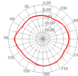
1900.000MHz E1
