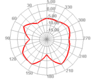
2450.000MHz E2
