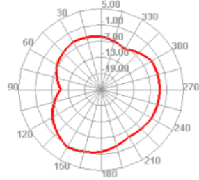
2400.000MHz H
