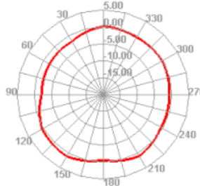
2100.000MHz E1
