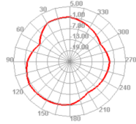
1700.000MHz E2
