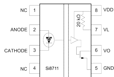
SOIC-8, DIP8
