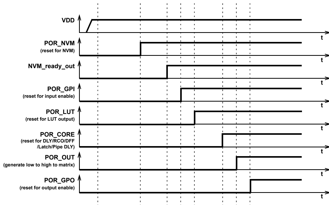
Figure 73. POR sequence
