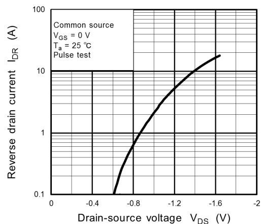
Fig. 8.8 I_{DR} - V_{DS}
