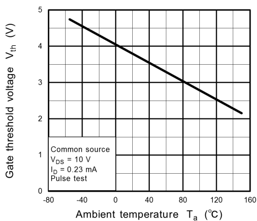
Fig. 8.11 V_{th} - T_a
