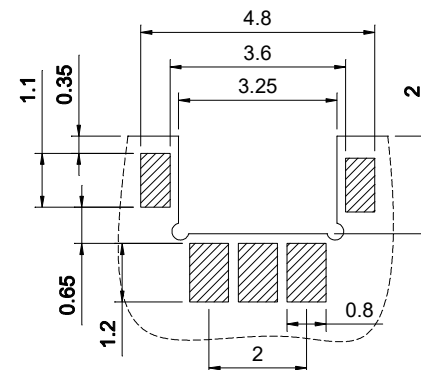
PCB. 焊接图
