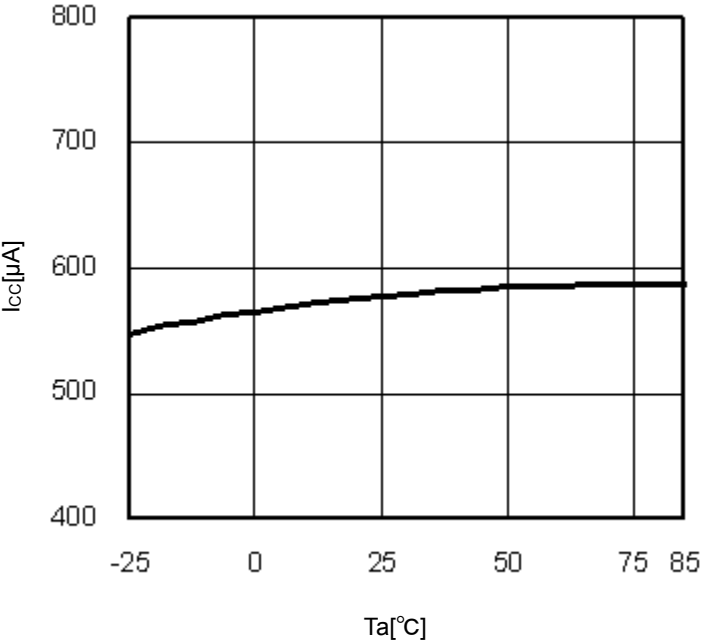
Fig.10 Ta-Icc
