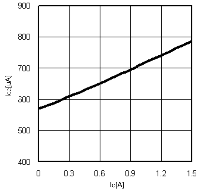
Fig.20 I_o - I_{cc}
