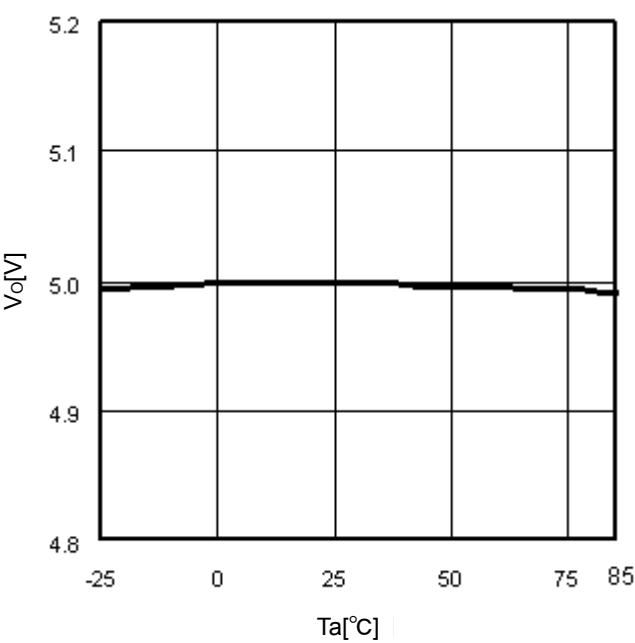
Fig.9 Ta-Vo (Io=0mA)
