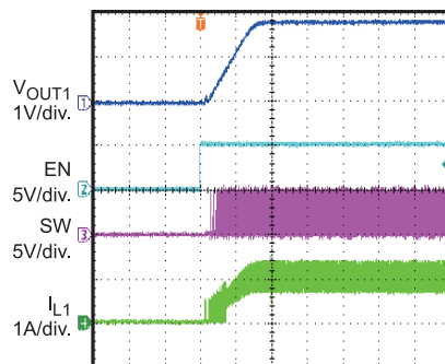
Enable On
