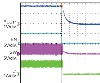
Enable Down
