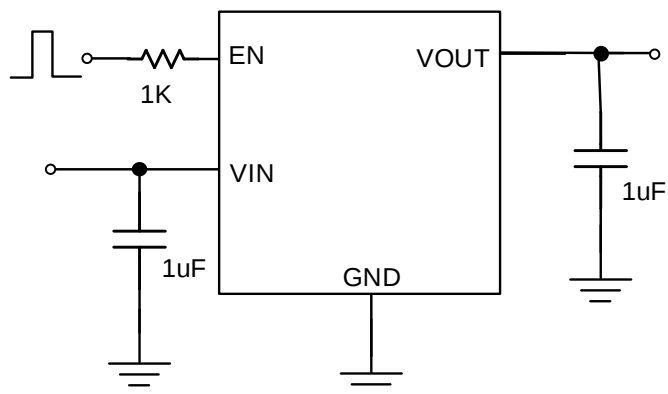
图：带使能脚的固定输出应用电路
