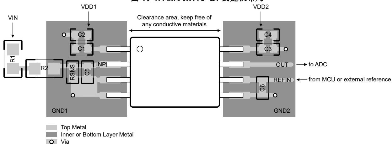
图 10-1. AMC0x11S-Q1 的建议布局
