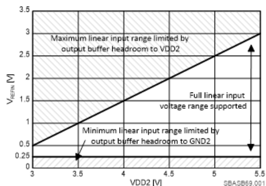
图 7-2. 线性运行的建议基准电压范围
