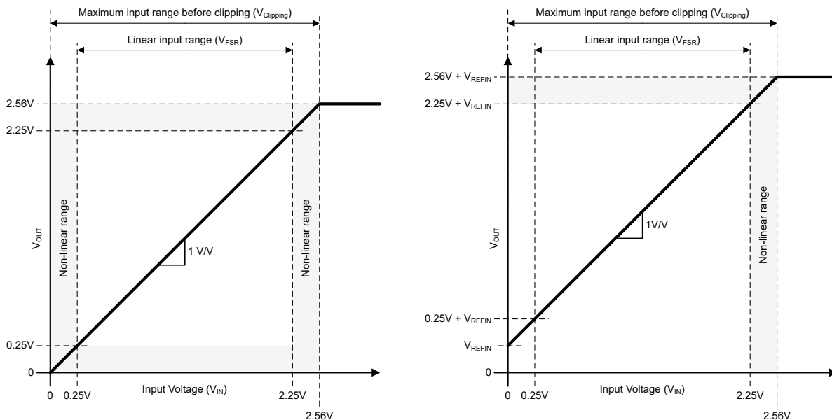
图 7-3. AMC0x11S-Q1 的输入到输出传递曲线 左：REFIN 短接至 GND2。右： V_{\text{REFIN}} = 250\text{mV}
