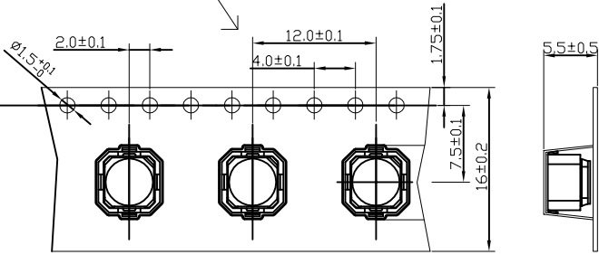
图2 成品盘带
