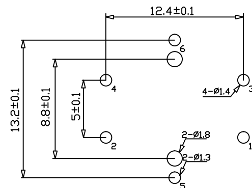
PCB线路板图
