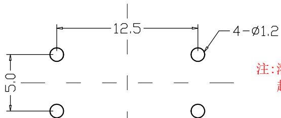
PCB线路板图
