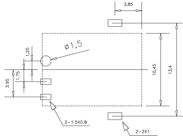
线路板安装尺寸示意图
