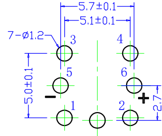
线路板图
