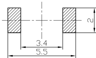
安装参考尺寸
