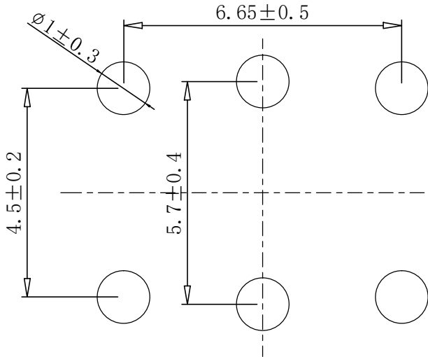
推荐PCB线路板图
