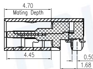
SECT A-A
