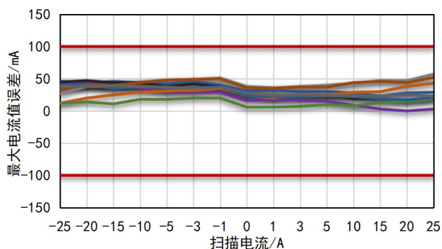
图 5-17. 105°C小电流测试精度@最大电流值误差
