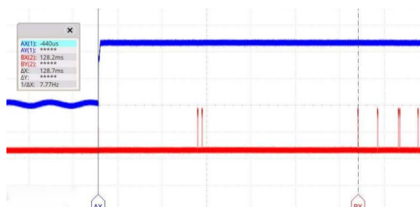
图 5-3. 样品 3 启动时间测试曲线
