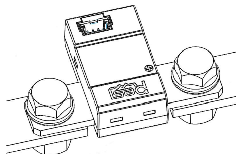
图 8-2. CB350M6918A1AA01_Y 铜排连接示意图
