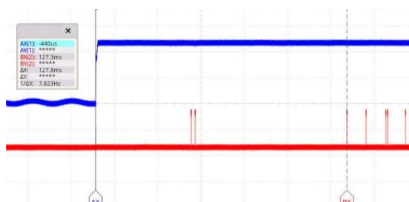
图 5-2. 样品 2 启动时间测试曲线
