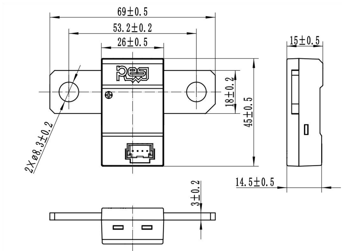
图 8-1. CB350M6918A1AA01_Y 电流传感器结构示意图
