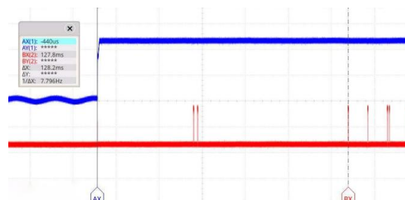
图 5-5. 样品 5 启动时间测试曲线
