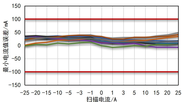
图 5-16. 105°C小电流测试精度@最小电流值误差
