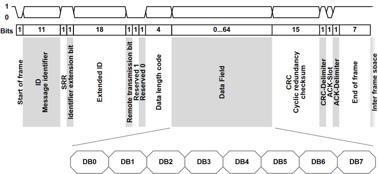
图 7-2. 扩展帧
