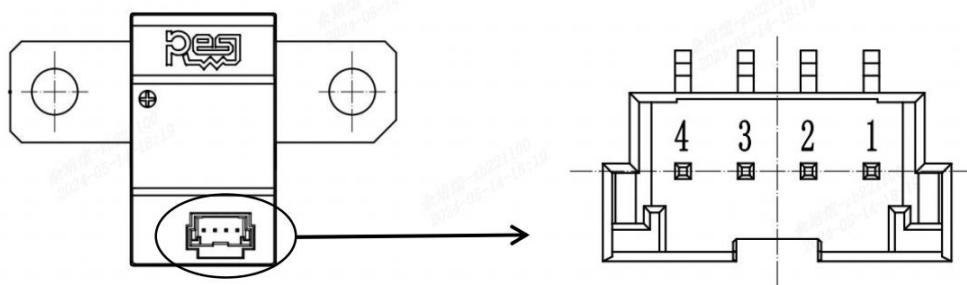
图 8-4. 公头连接器 Molex5600200420
