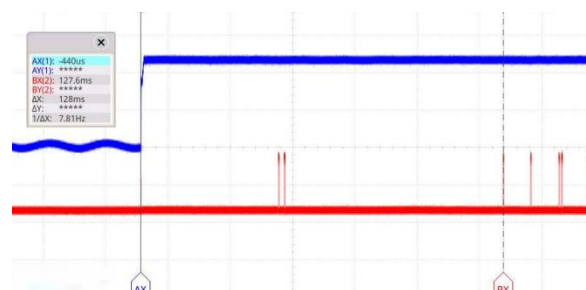
图 5-7. 样品 7 启动时间测试曲线
