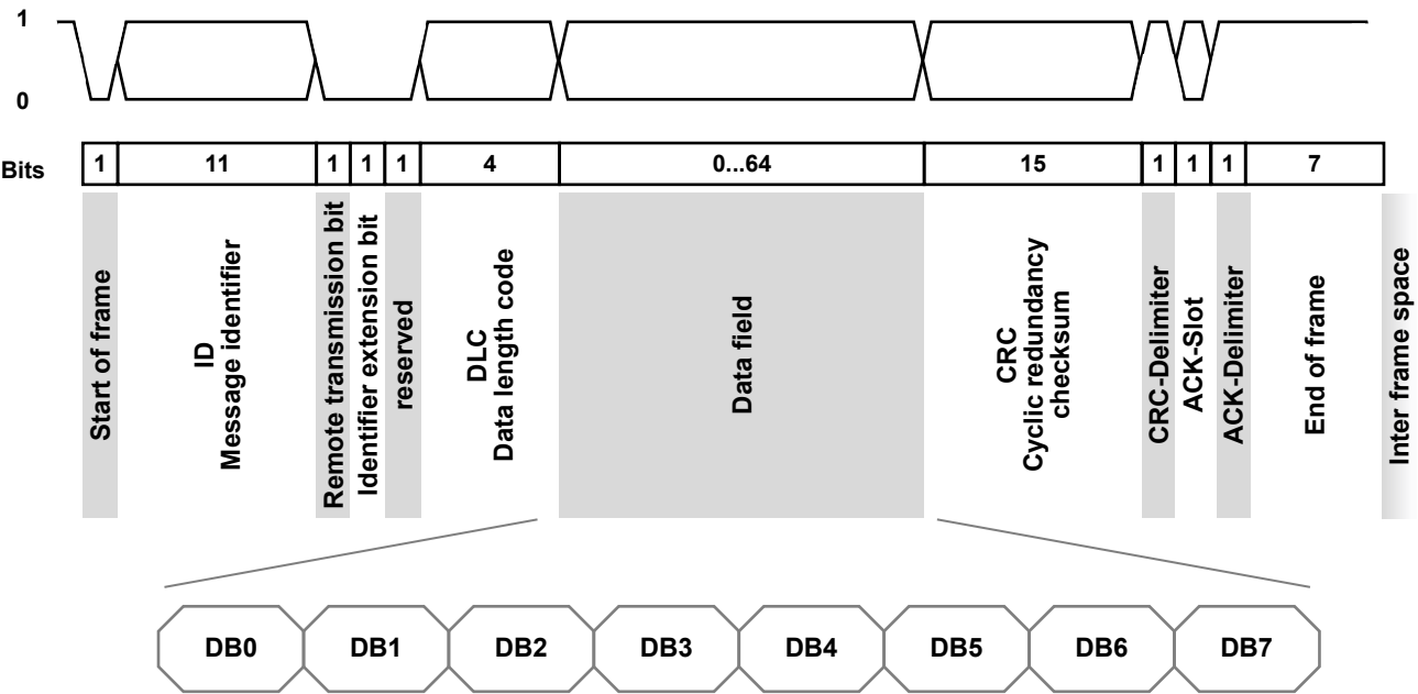
图 7-1. 标准帧
