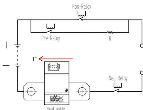
典型应用
