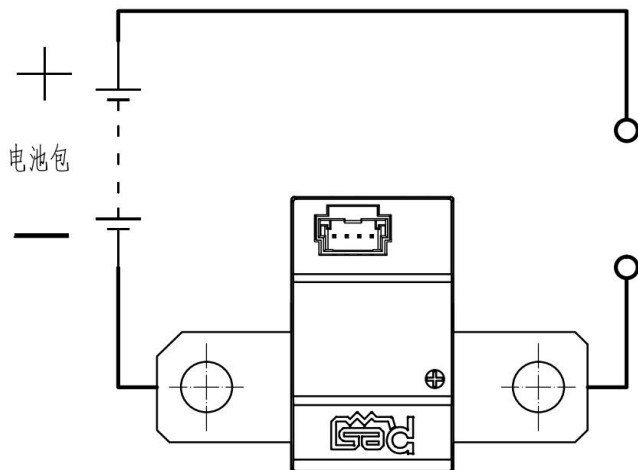
图 9-2. 高压主负端推荐使用场景
