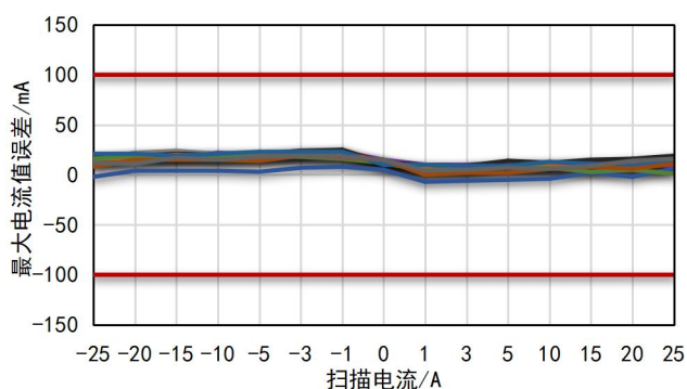
图 5-15. 25°C小电流测试精度@最大电流值误差
