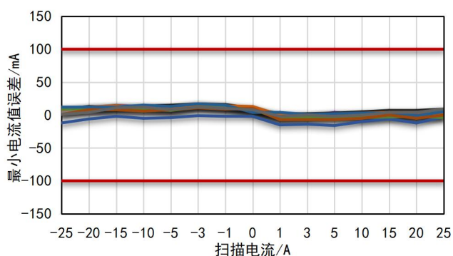
图 5-14. 25°C小电流测试精度@最小电流值误差
