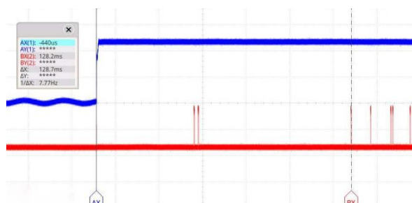
图 5-4. 样品 4 启动时间测试曲线
