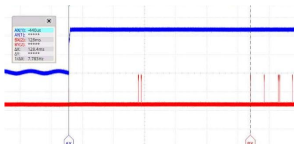
图 5-1. 样品 1 启动时间测试曲线
