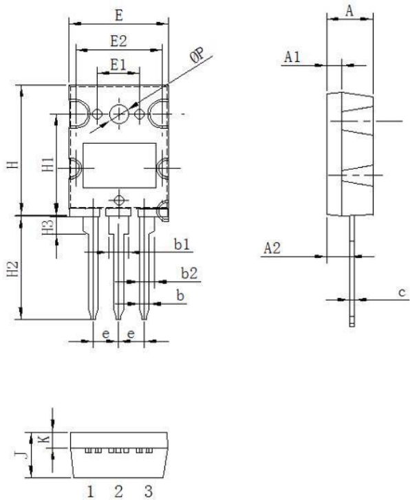
外形名称: TO-264
