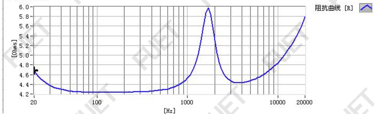
阻抗曲线
