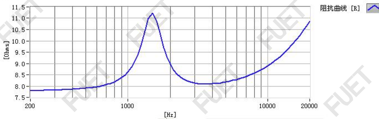
阻抗曲线
