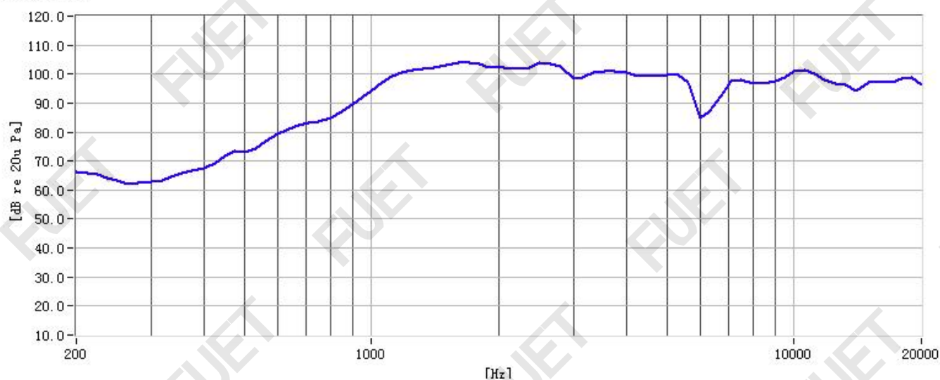
频响曲线
