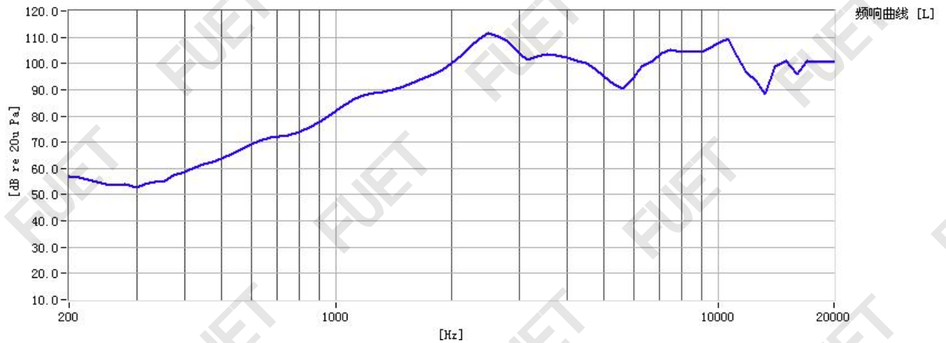
频响曲线
