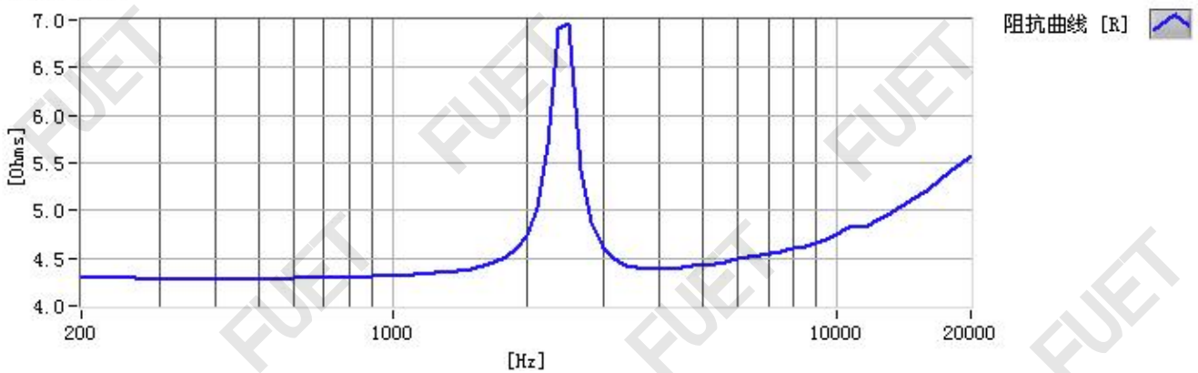
阻抗曲线
