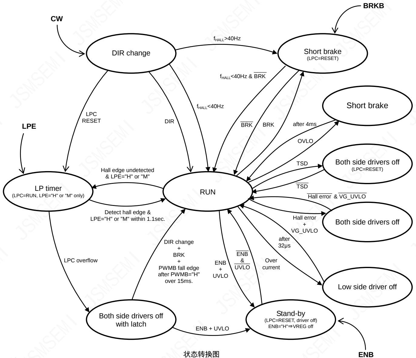
状态转换图
