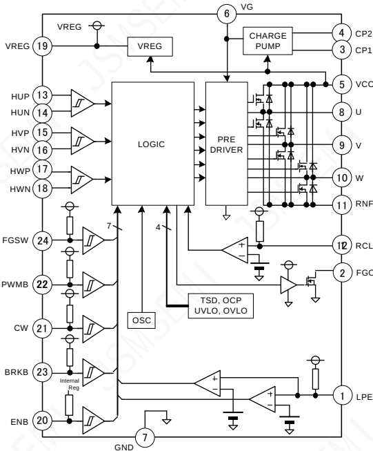
功能框图
