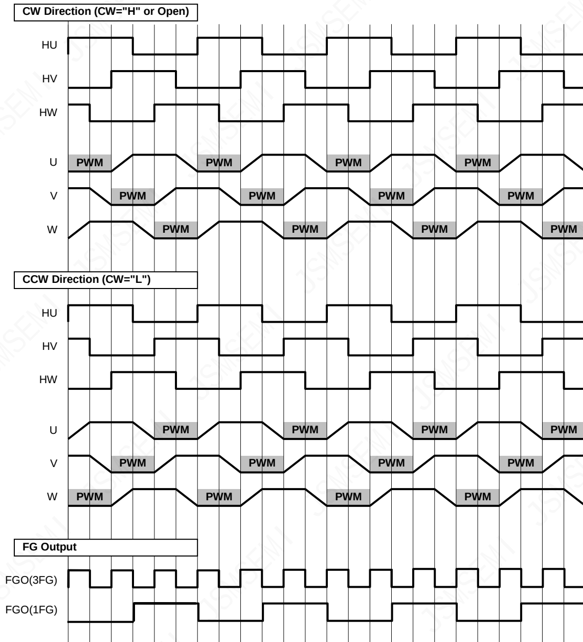
时序图
