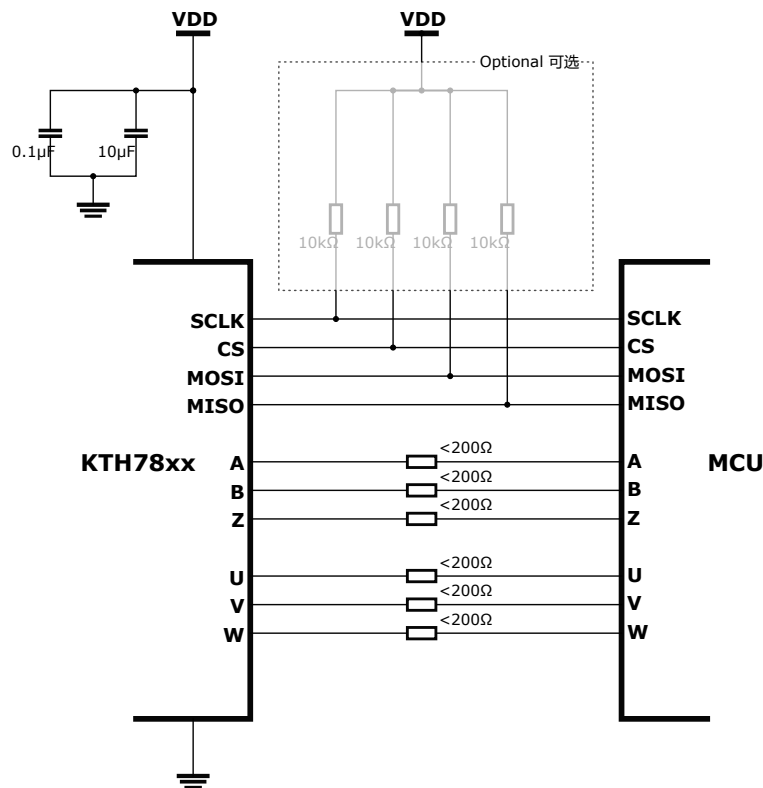
图 2: 应用电路
