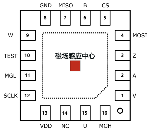
图 3: QFN-16L 3mmx3mm
