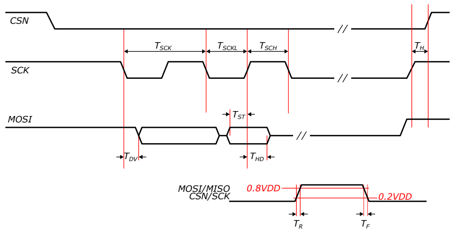
图 8: SPI 时序图
