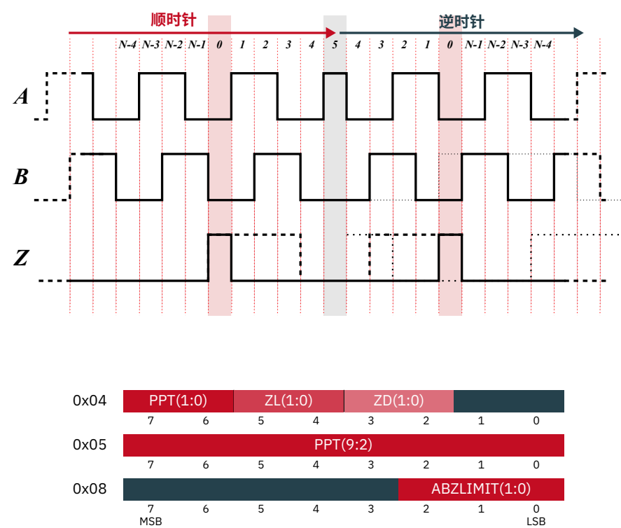
图 10: ABZ 输出时序
