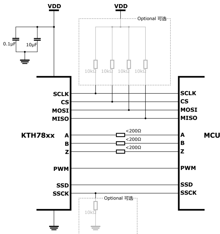
图 2: 应用电路
