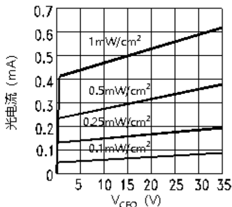
图六：光电流VS VCE曲线
