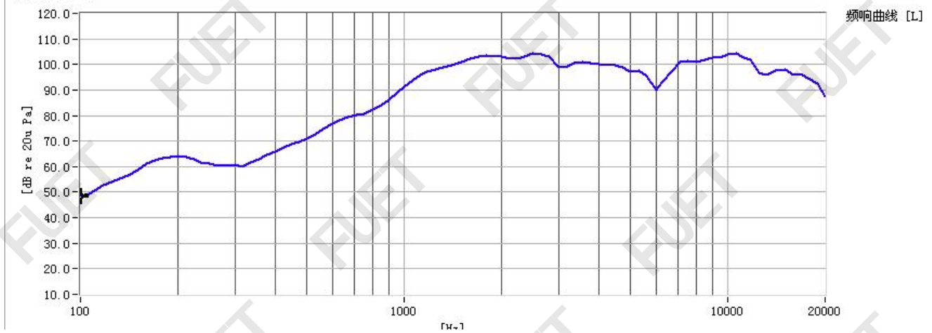
频响曲线
