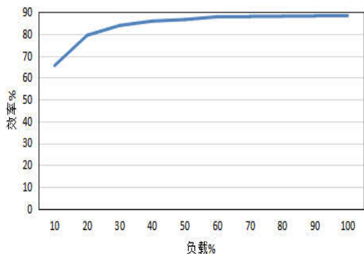
12V 输出典型效率曲线图
