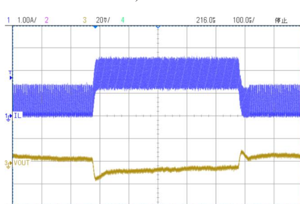
(15) 负载瞬变(输入电压 15.0V, 输出电压 3.3V, 负载电流 0.5→1.8A)
