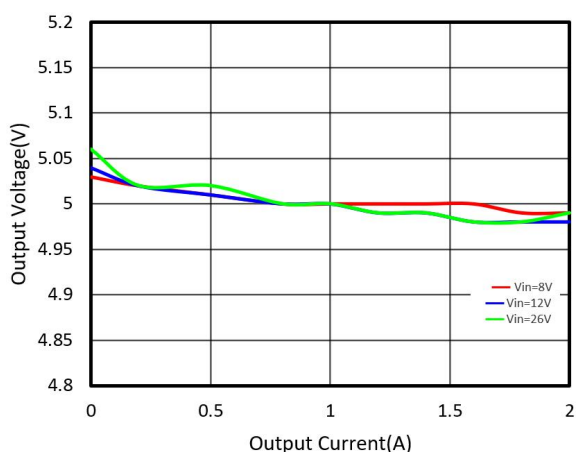
(4)输出电压与负载电流(输出电压 5.0V)
