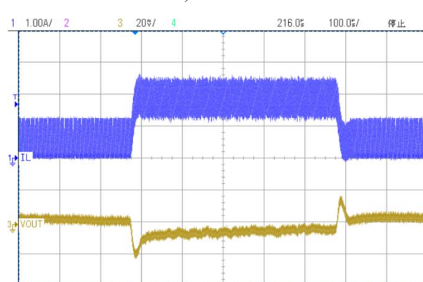
(16) 负载瞬变(输入电压 15.0V, 输出电压 5.0V, 负载电流 0.5→1.8A)
