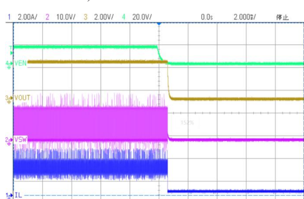
(18) EN 关断(输入电压 15.0V, 输出电压 3.3V, 负载电流 2A)
