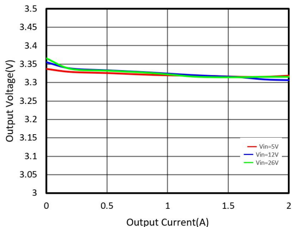
(3)输出电压与负载电流(输出电压 3.3V)
