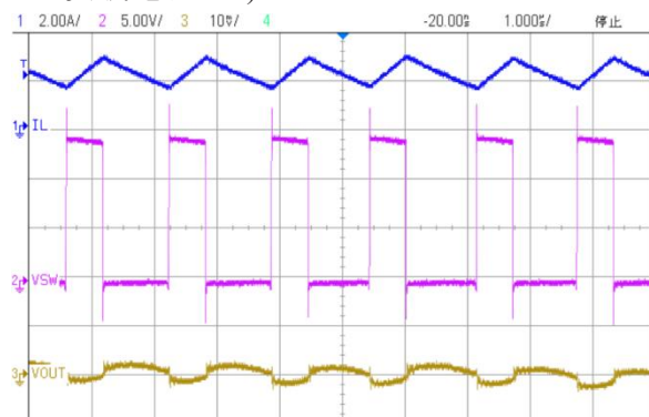
(14) 输出纹波(输入电压 15.0V, 输出电压 5.0V, 负载电流 2A)
