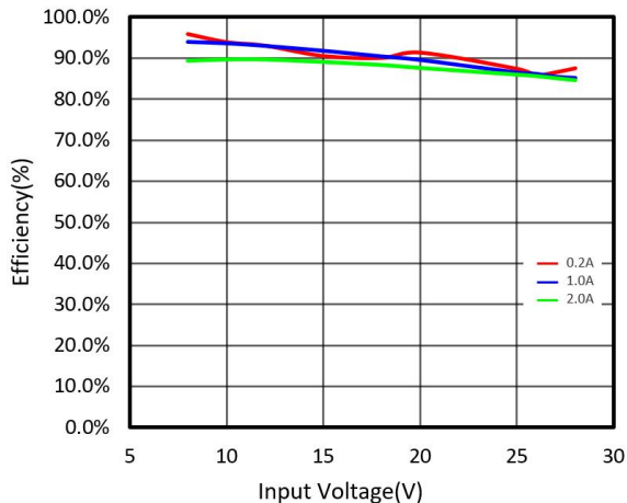
(10) 转化效率与输入电压(输出电压 5.0V)
