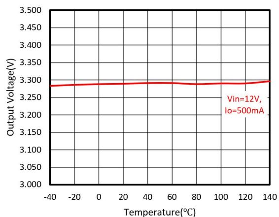
(11) 输出电压与温度(输出电压 3.3V)
