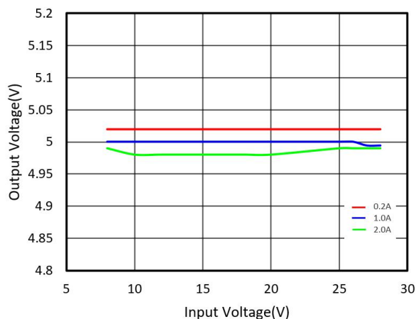
(6)输出电压与输入电压(输出电压 5.0V)
