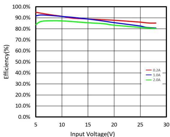
(9) 转化效率与输入电压(输出电压 3.3V)
