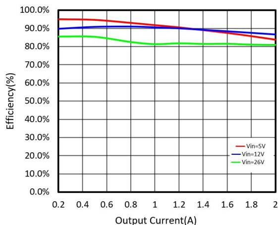
(7) 转化效率与负载电流(输出电压 3.3V)
