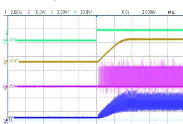
(17) En 启动(输入电压 15.0V, 输出电压 3.3V, 负载电流 2A)
