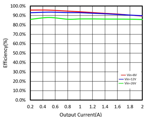
(8) 转化效率与负载电流(输出电压 5.0V)
