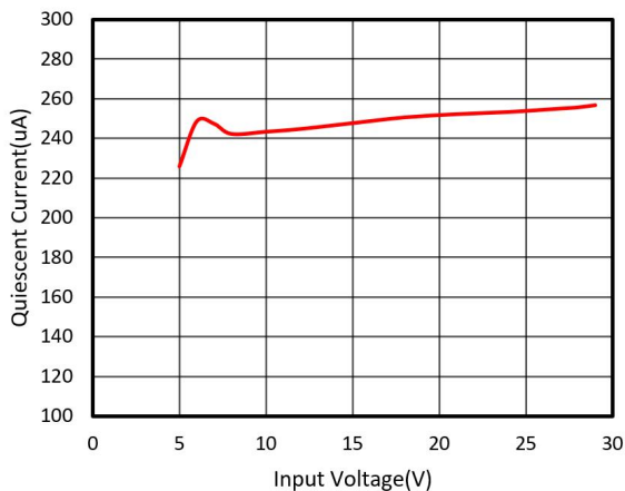
(1)静态电流与输入电压
