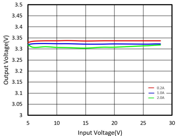
(5)输出电压与输入电压(输出电压 3.3V)
