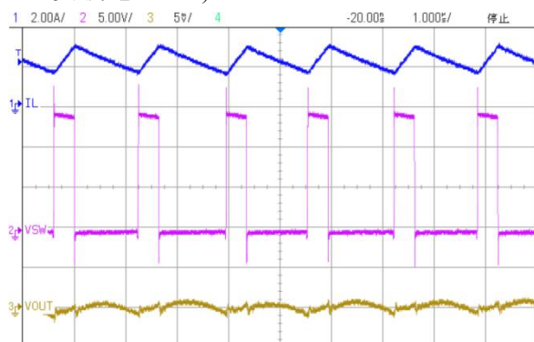
(13) 输出纹波(输入电压 15.0V, 输出电压 3.3V, 负载电流 2A)
