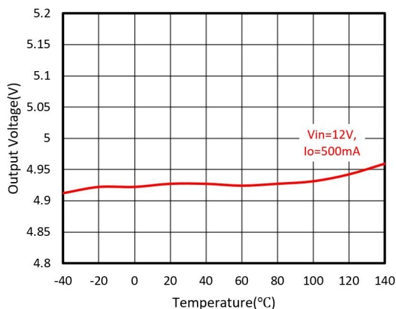
(12) 输出电压与温度(输出电压 5.0V)
