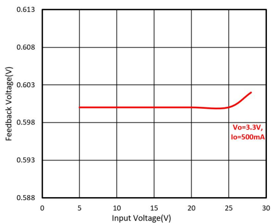
(2)反馈电压与输入电压
